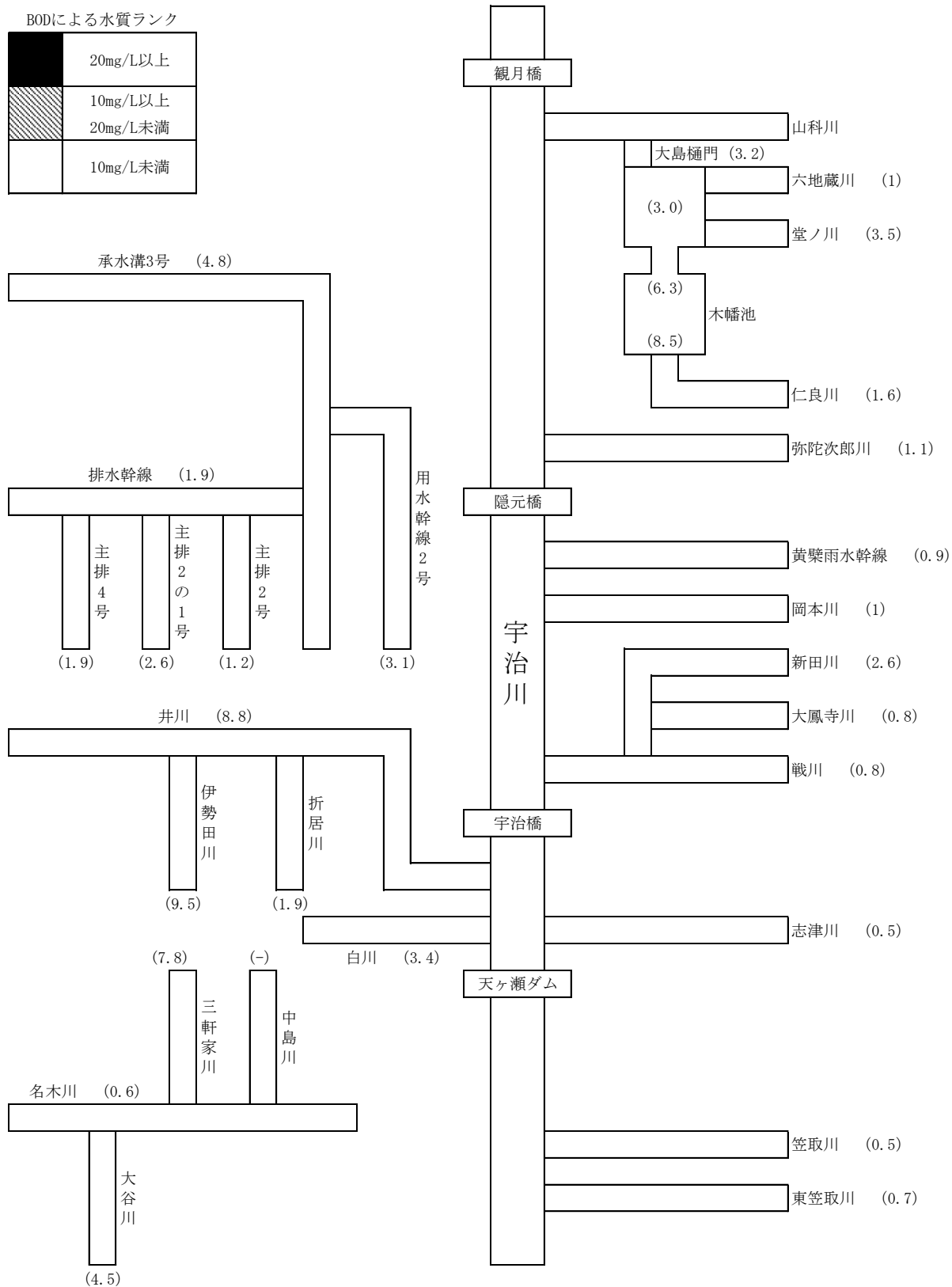
図 4-2-1 市内河川汚濁状況図（令和 5 年度）
