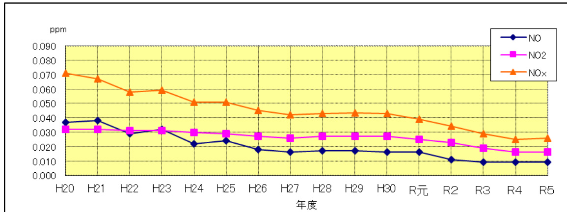
図4-5-2 窒素酸化物の経年変化（年間98%値）
