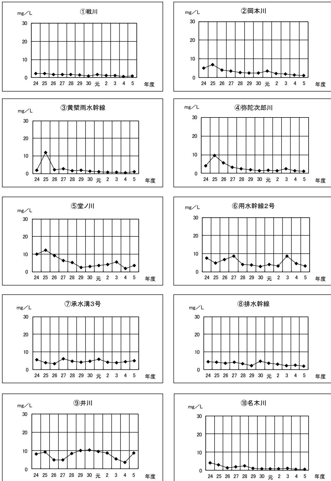
図4-2-3 中小河川水質（BOD 値）の経年変化
