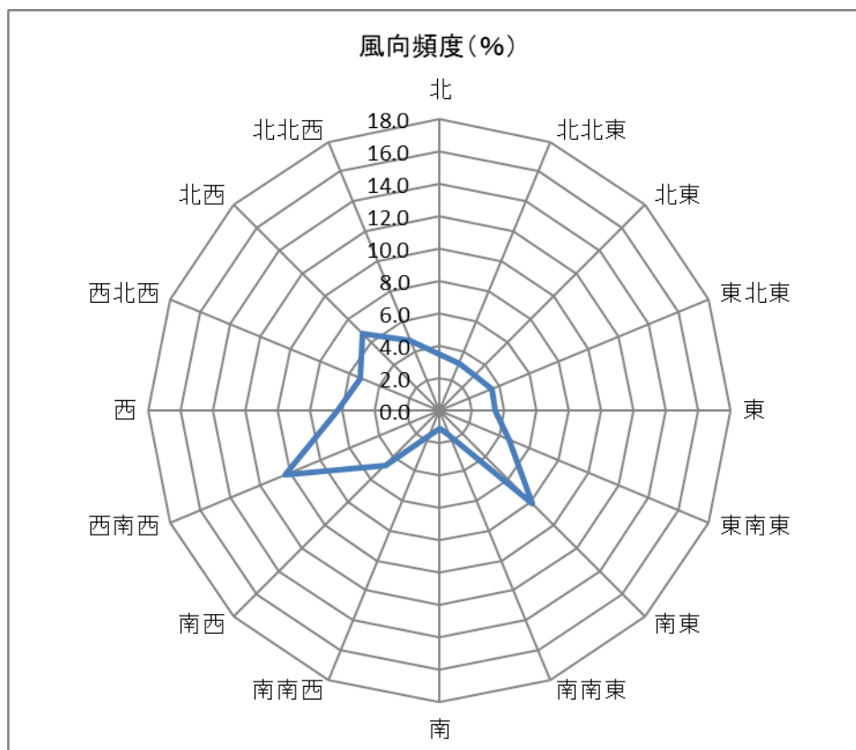
図4-5-6 令和5年度福角局風配図
