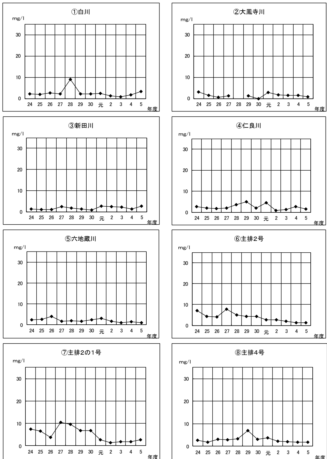
図 4-2-4 生活系支川・水路水質（BOD 値）の経年変化
