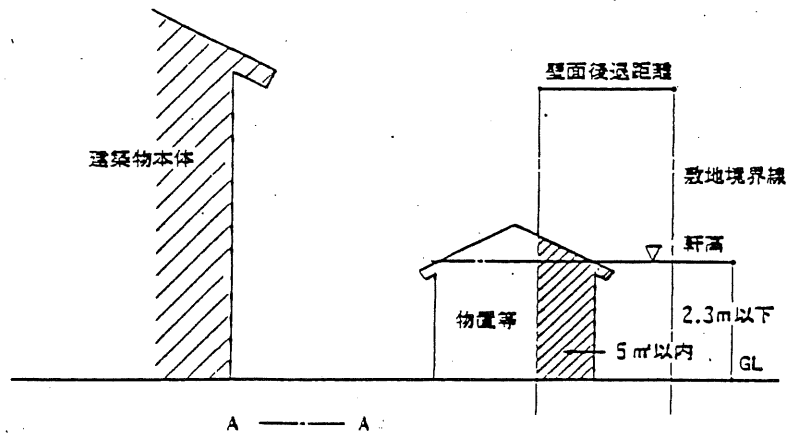
断面図
