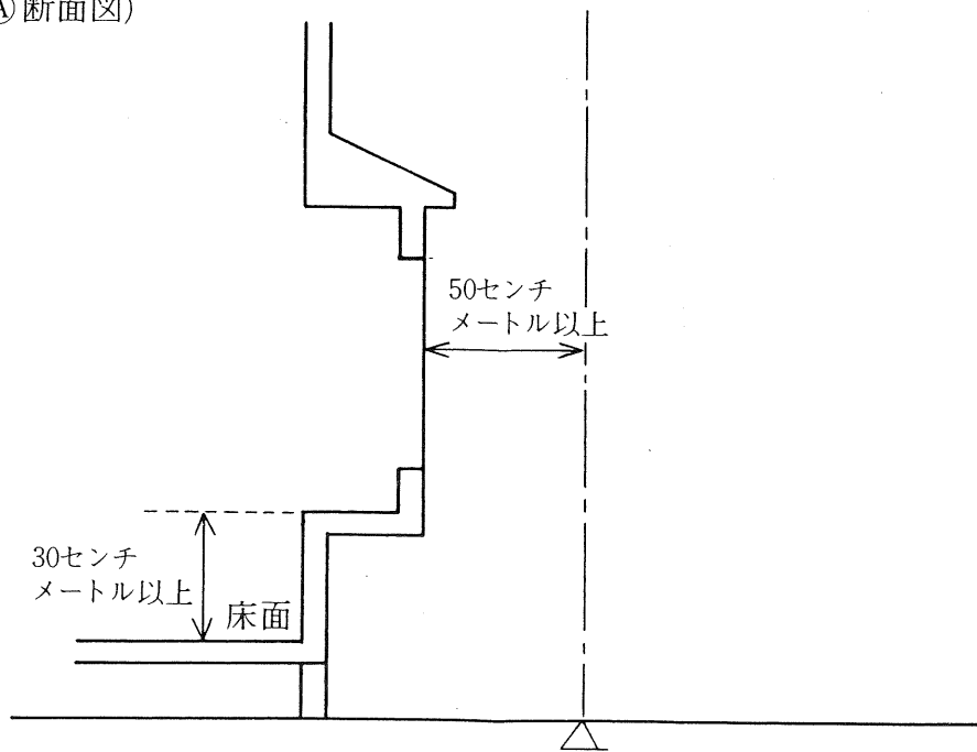
(A-A断面図)
