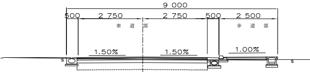
標準断面図
