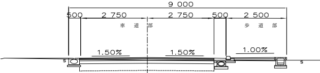
標準断面図
