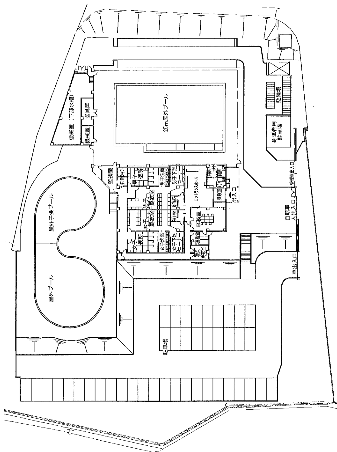
黄檗公園プール 平面図
