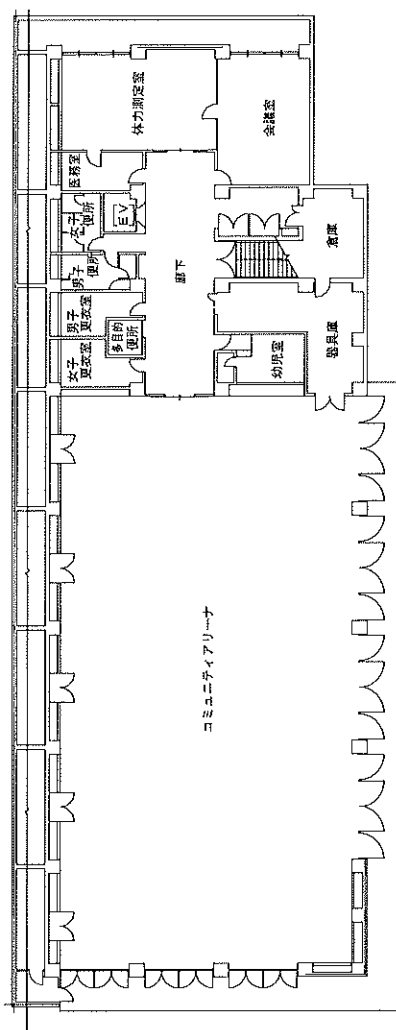
黄檗公園体育館 1 階
