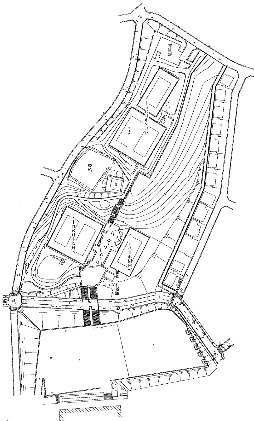
東山公園平面図
