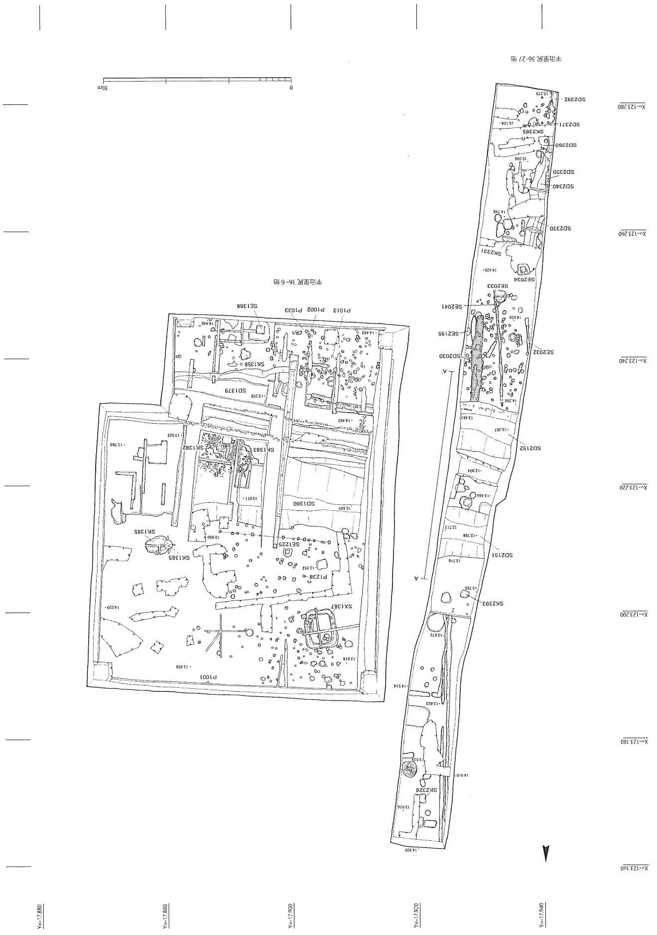
図面図版 6 トノチ平面実測図(下層面)
