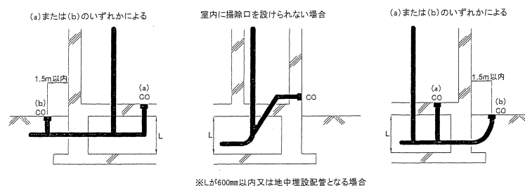
掃除口設置位置の例
