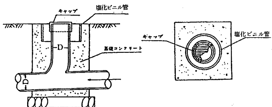
掃除口設置例
