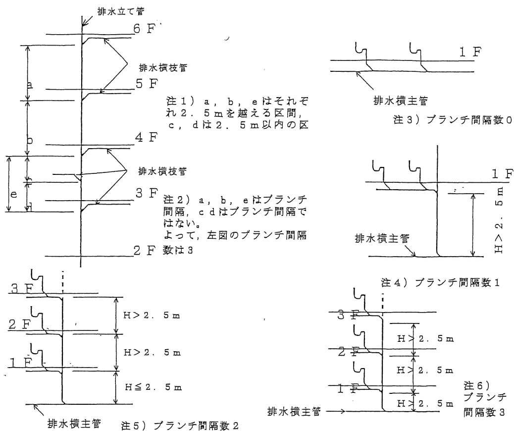
図 2-3 ブランチ間隔数の考え方
