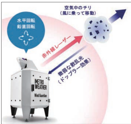
▲ドップラー・ライダーの動作原理
