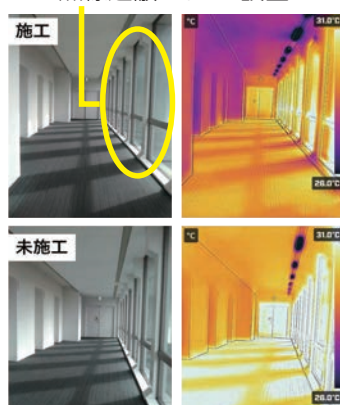
▲熱線遮蔽フィルムの実証実験
