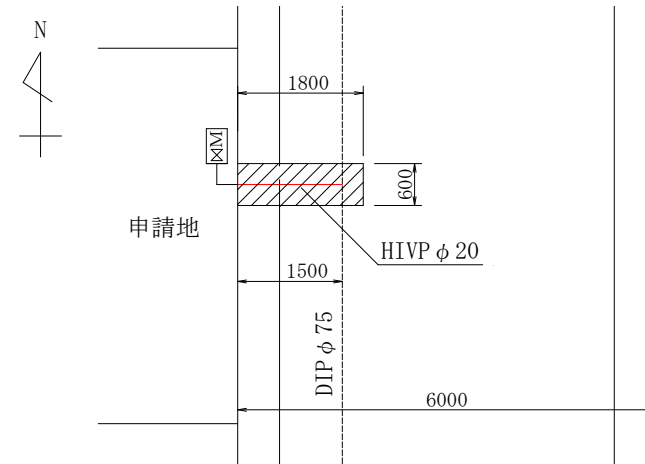
平面図 S=1:100
