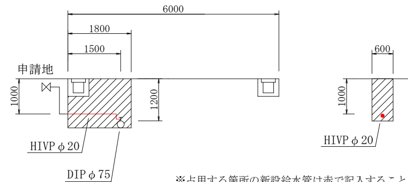
断面図 S=1:100
