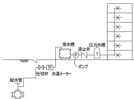
圧力水槽式
