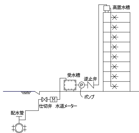
高置水槽式
