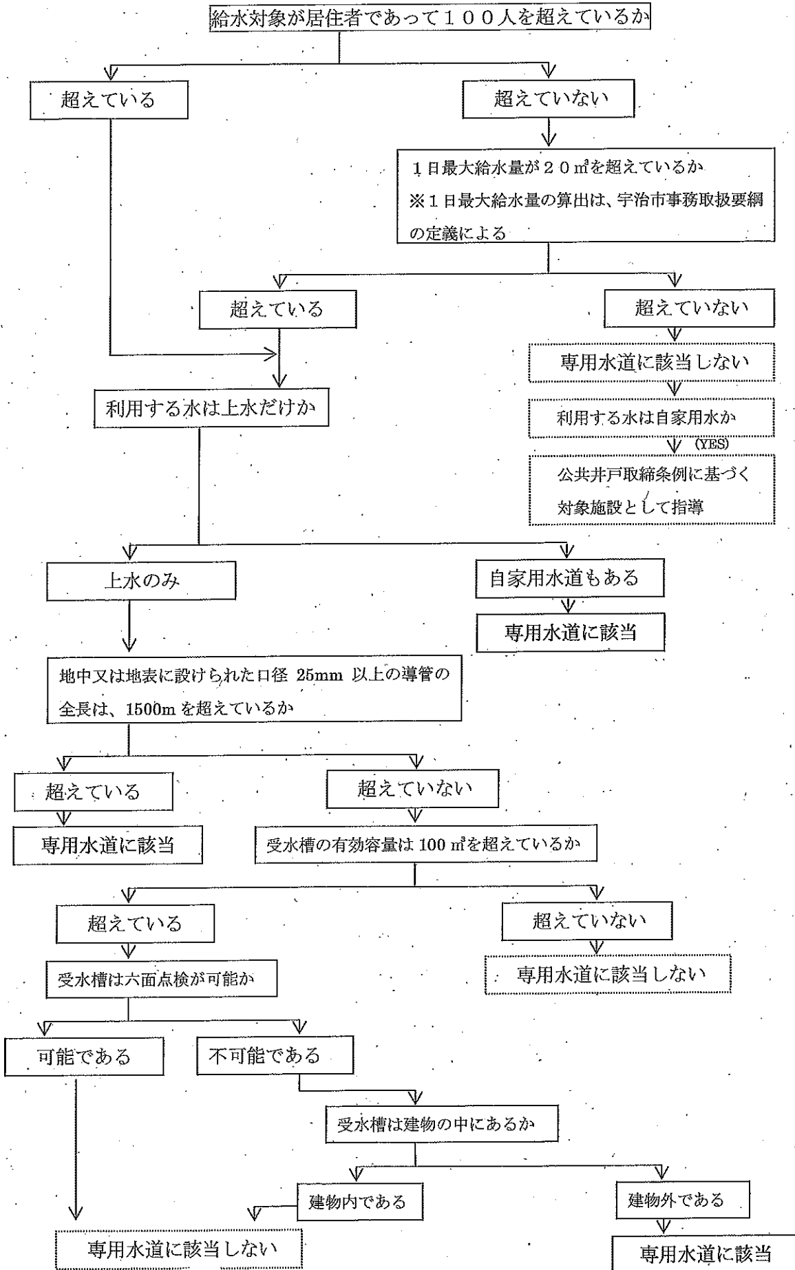
宇治市専用水道事務取扱要項における専用水道の定義略図
