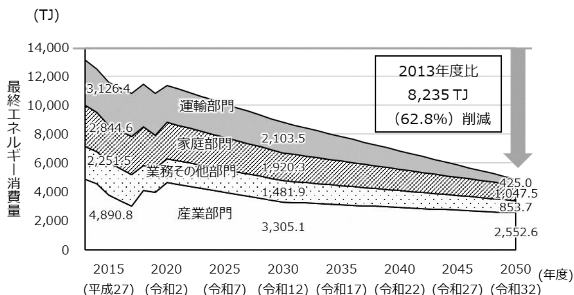
図 資 2-19 【エネルギー消費量(脱炭素シナリオ)の推移】
