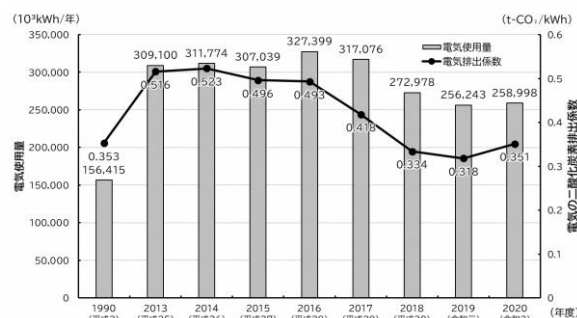
図資2-13 【業務その他部門の電気使用量及び二酸化炭素排出係数の推移】
