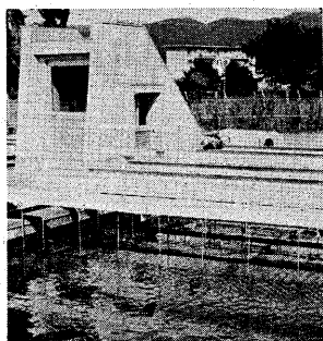
▲薬品沈殿池新設工事が行われる宇治浄水場
