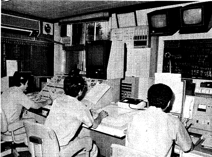
指令室に設置された緊急情報現示システム (中央のブラウン管に市街地図などが映る)
