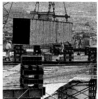
◀宇治川をまたぐ橋げた(1月27日)
