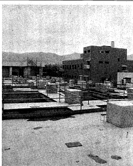
▲東宇治下水処理場の管理棟(右)と沈殿池(手前) (8月23日)
