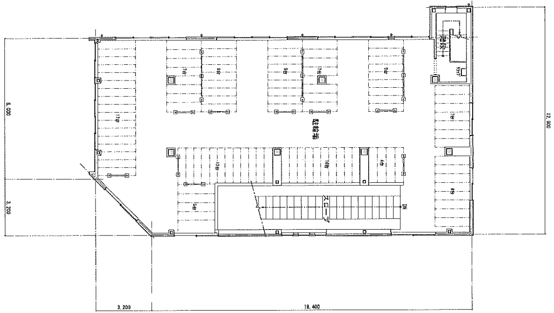
3 层平面图
