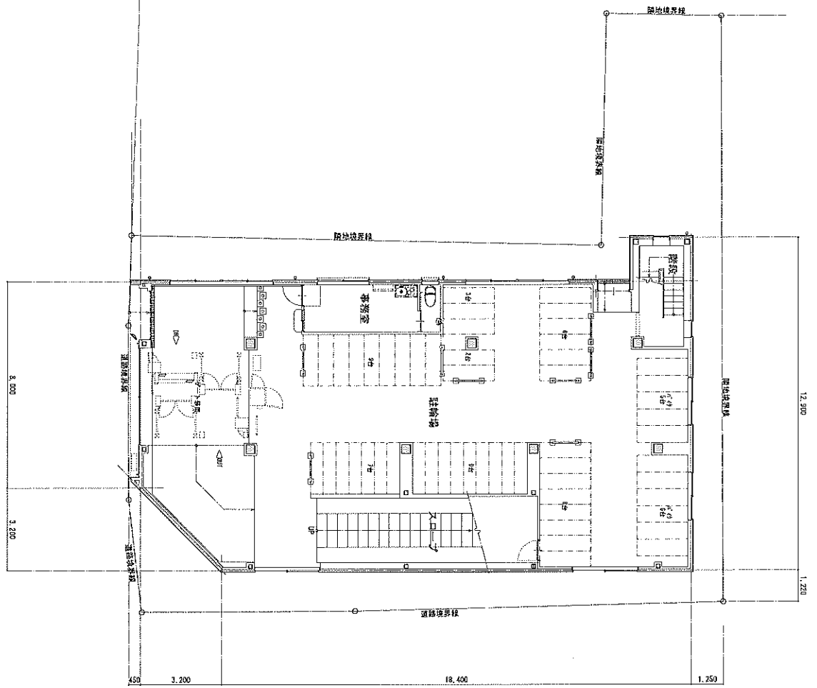
1 层平面图
