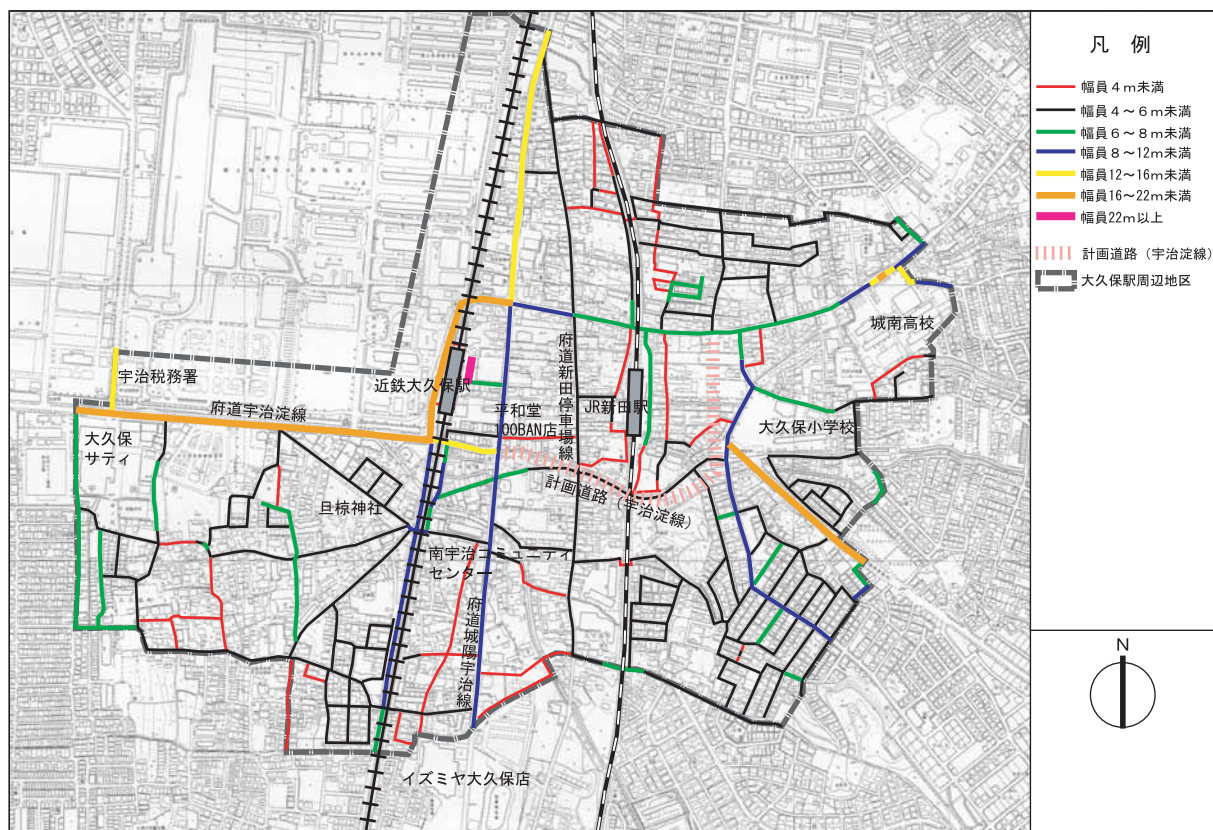
図2-3 幅員別道路現況図
