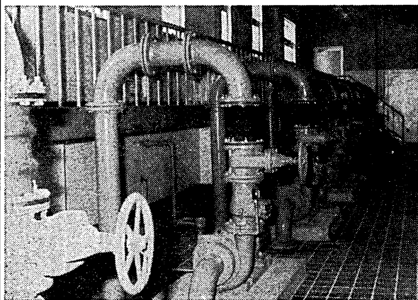
ろ過ポンプ 薬品処理された水を 急速ろ過装置に送り ます
