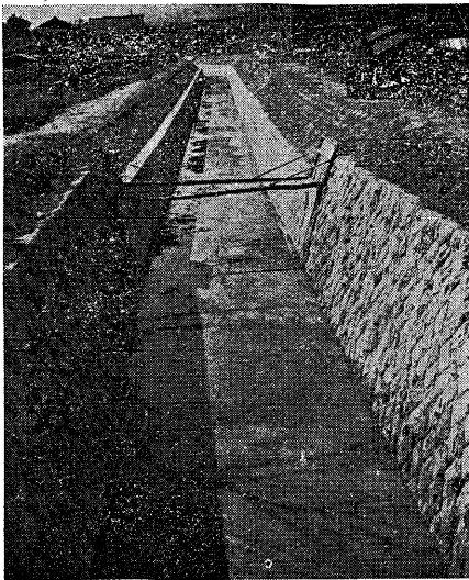
一部完成した堂の川災害関連工事（木橋上流から）
