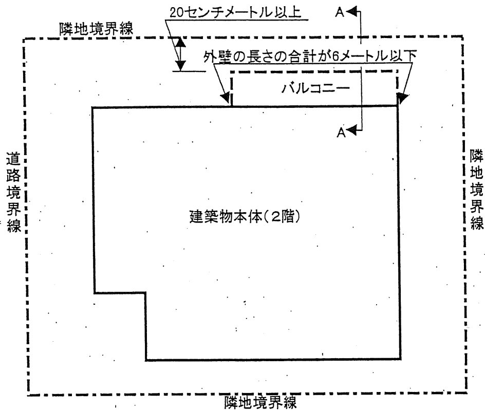
A-A断面
