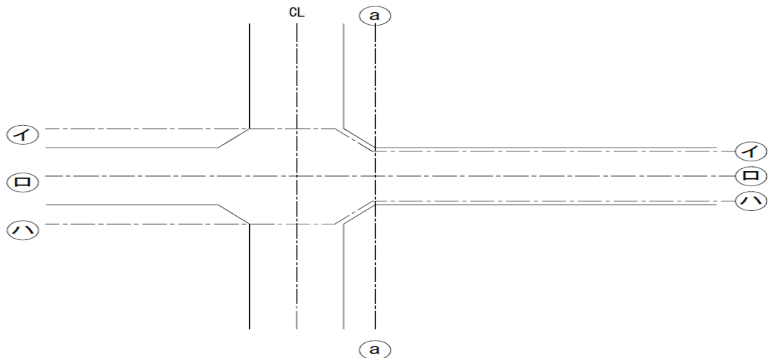
図-4 (取付け先道路に勾配がある場合)
